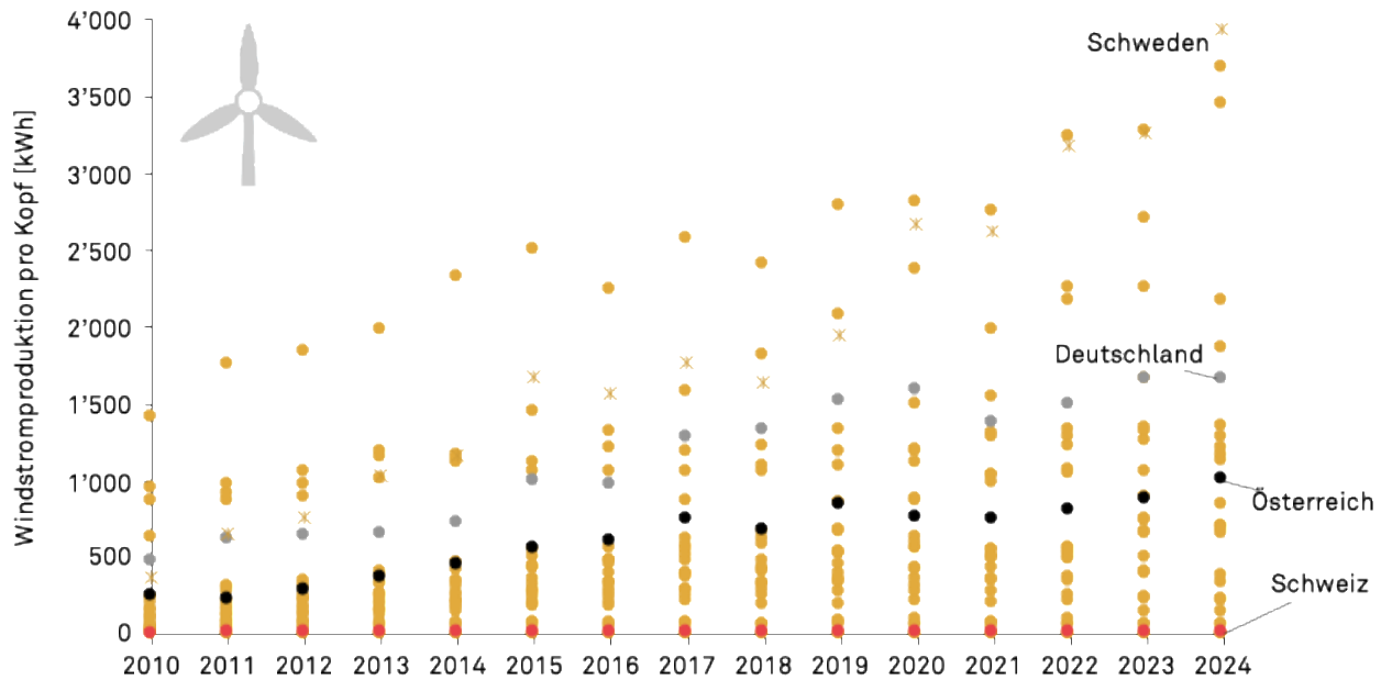
Abbildung 2. Ausbau der gesamten Solar- und Windstromproduktion pro Kopf (a) und nach aufgeteilt nach Technologie (Solar, b und Wind, c) von 2010 bis 2024 in der Schweiz (rot), Deutschland (grau), Österreich (schwarz) und dem jeweiligen führenden Land (Stern), sowie den übrigen EU-Staaten. Daten bis 2023 aus den früheren Ländervergleichen der SES.
