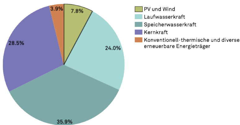
Abbildung 1. Schweizer Stromproduktion 2024 nach Energieträger. Daten: BFE 2025, Suisse Eole 2025a, Swissolar 2024, eigene Berechnungen. Eigene Darstellung.
